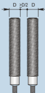
Montaggio affiancato
